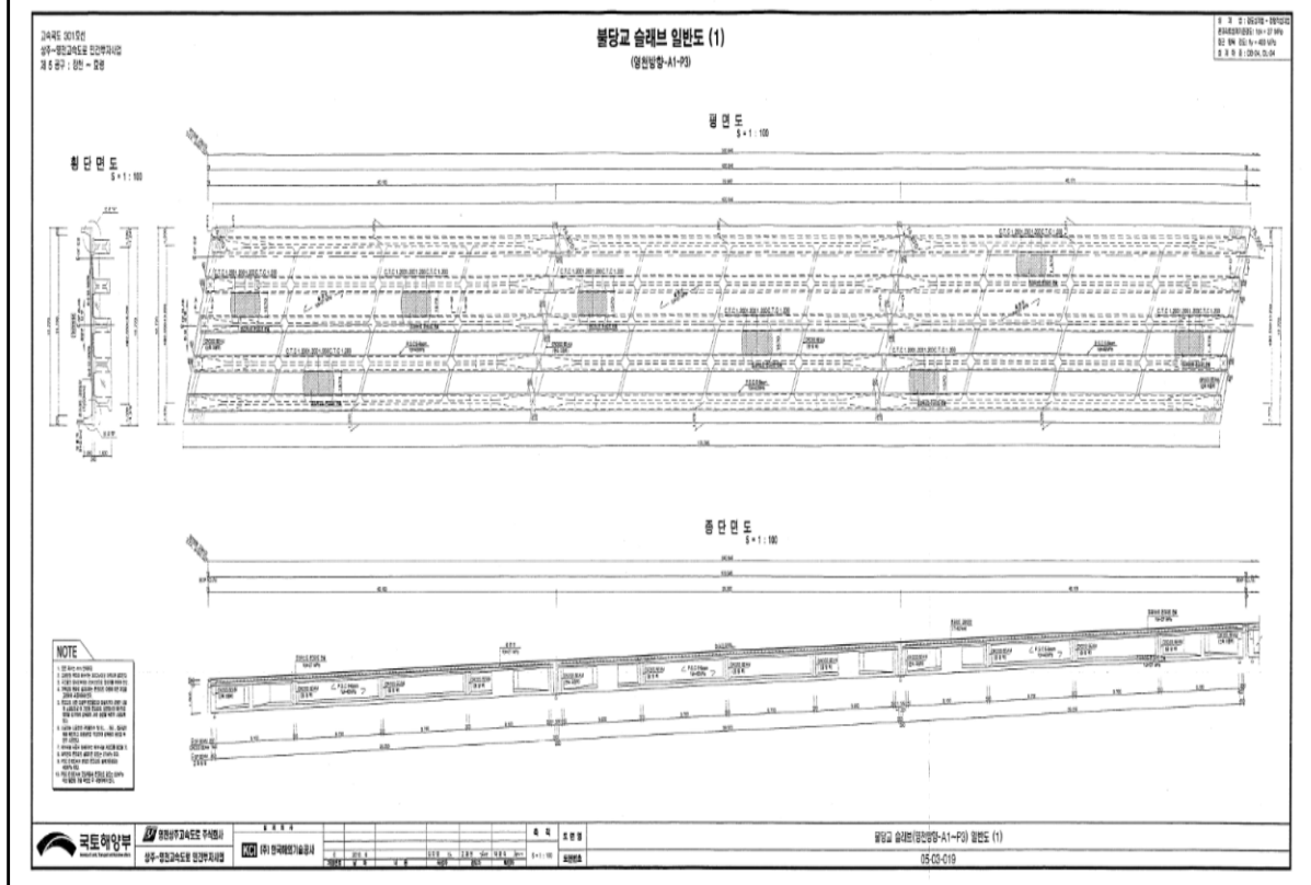
【그림 11.1.4】 슬래브 일반도
