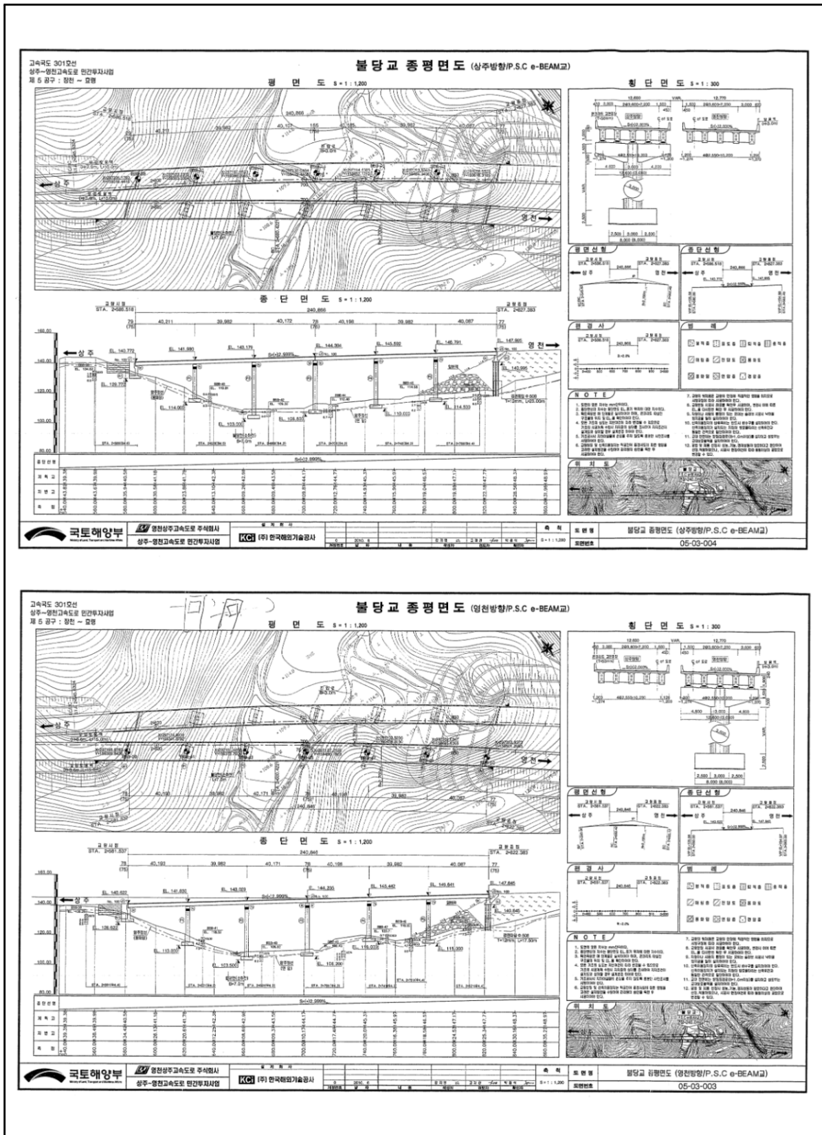
【그림 11.1.3】 종평면도
